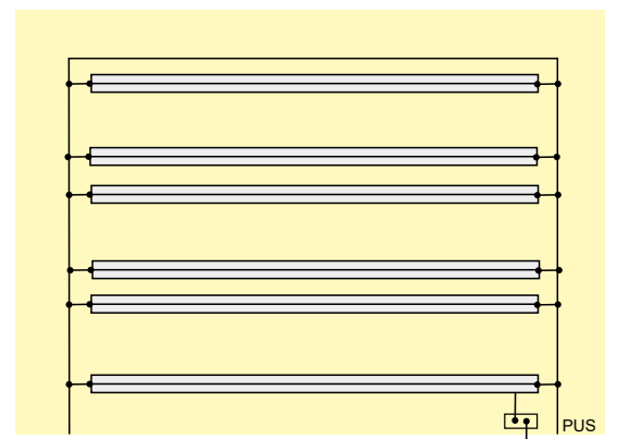
Potentialutjämning av ramverk, där man inte upprätthåller skiljeavstånd.
