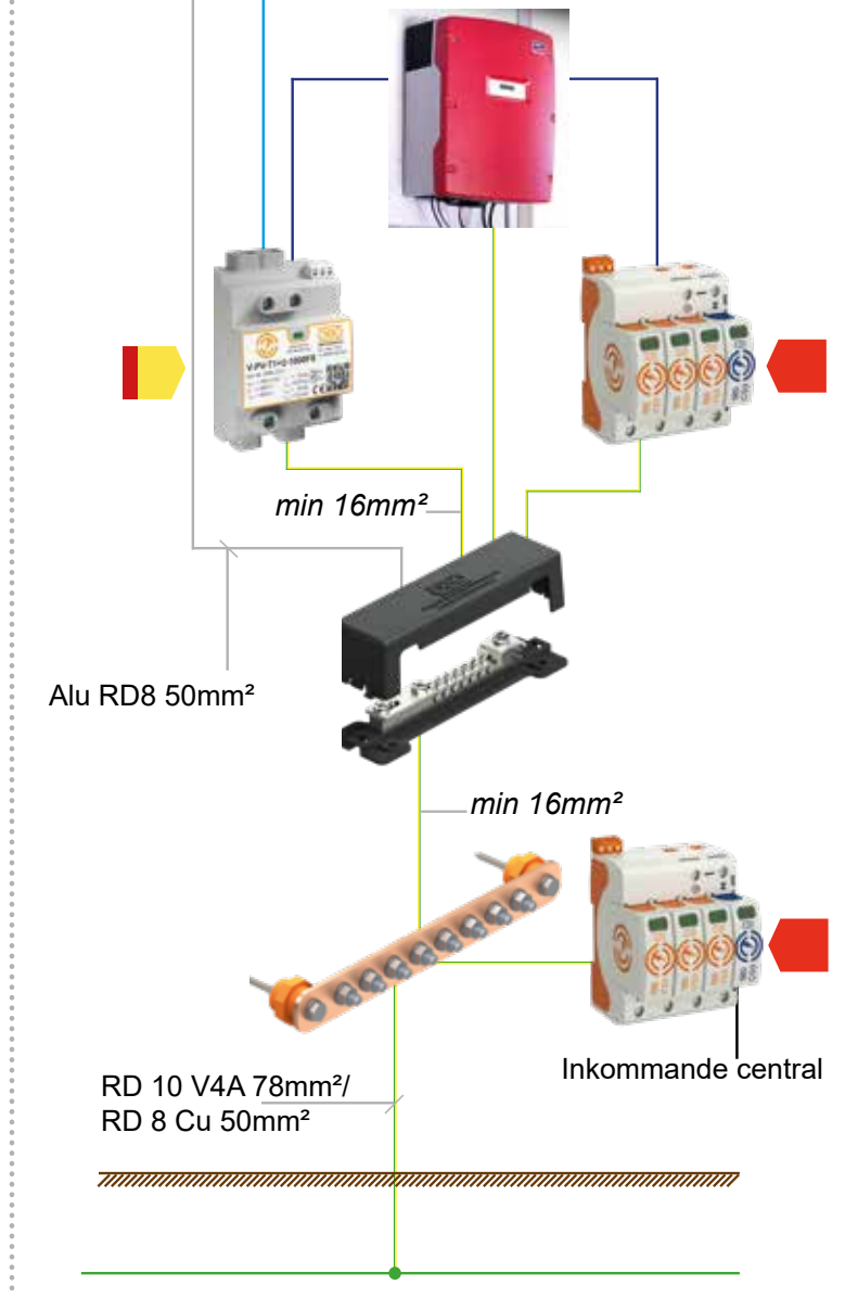
Potentialutjämning av ramverk, där man inte upprätthåller skiljeavstånd.
